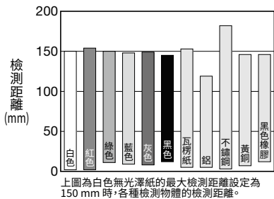
●顏色 (100×100mm 無光澤紙)、材質—檢測距離特性 (150mm時)
