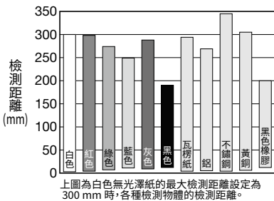
●顏色 (100×100mm 無光澤紙)、材質—檢測距離特性 (300mm時)
