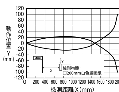
●動作範圍特性
