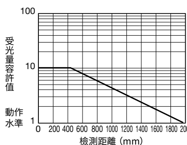
●受光量—檢測距離特性
