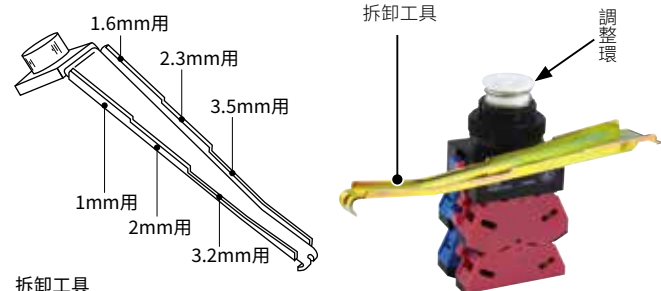
拆卸工具
