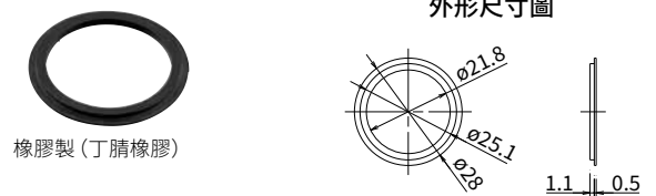
外形尺寸圖
