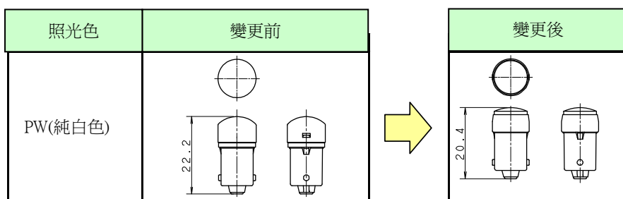
圖 1. LED 燈泡形狀變更
