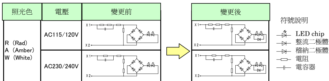
圖 2.內部回路變更
