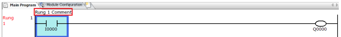
圖 3: 下載的程式
